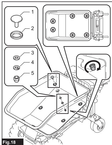
► 1. Perno 2. Arandela de goma 3. Arandela plana 4. Arandela de muelle 5. Tuerca
