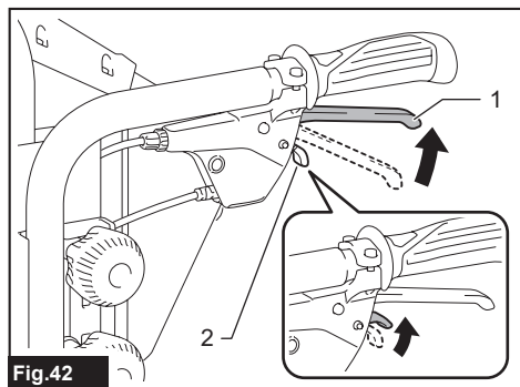
Fig.42 ► 1. Palanca del freno 2. Palanca de bloqueo
