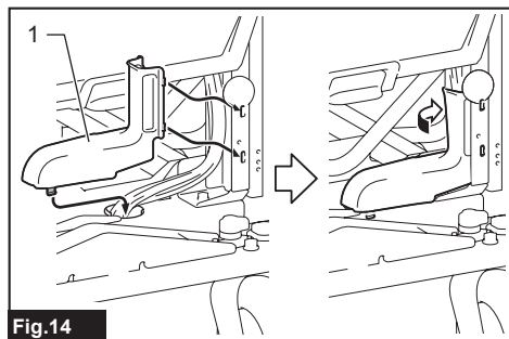
► 1. Cubierta del cable
