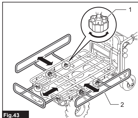
► 1. Thumb nut 2. Rail
