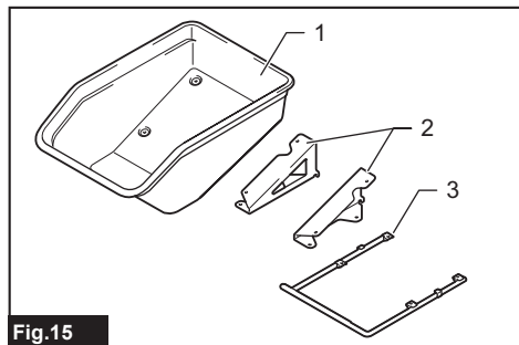
► 1. Canasta 2. Retenedor 3. Tubo frontal
